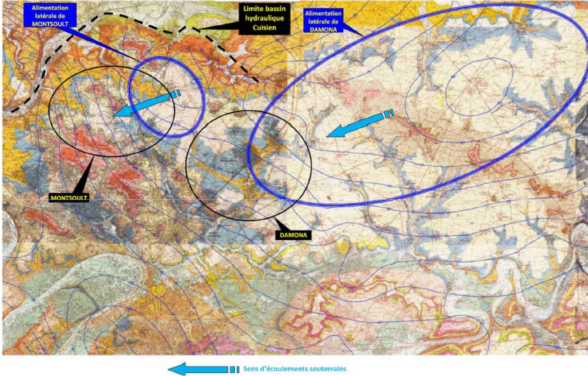
Étendue des zones d'alimentation latérale dans la nappe des sables cuiens
