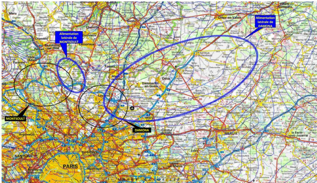
Étendue des zones d'alimentation latérale dans la nappe des sables cuiens
